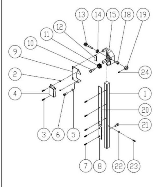
Detailzeichnung zu Nr. 176
