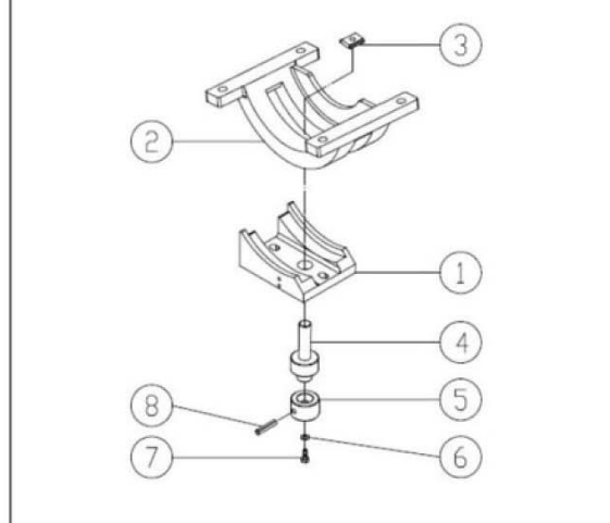
Detailzeichnung zu Nr. 147
