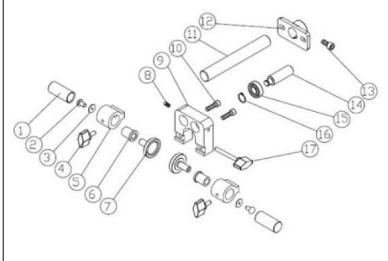
Detailzeichnung zu Nr. 229
