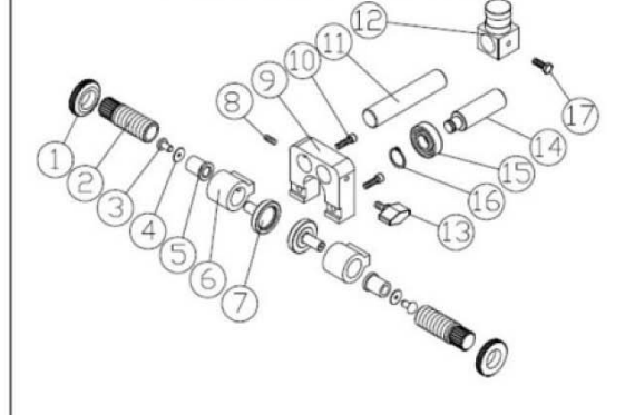
Detailzeichnung zu Nr. 230
