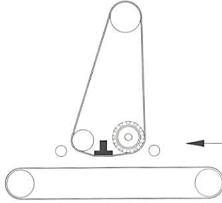
Feinschleifen mit dem Schleifschuh
