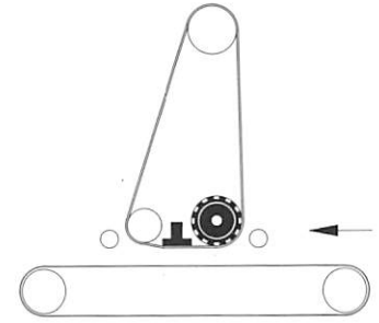
Combischliff mit Kontaktwalze und zusätzlichem Schleifschuh
