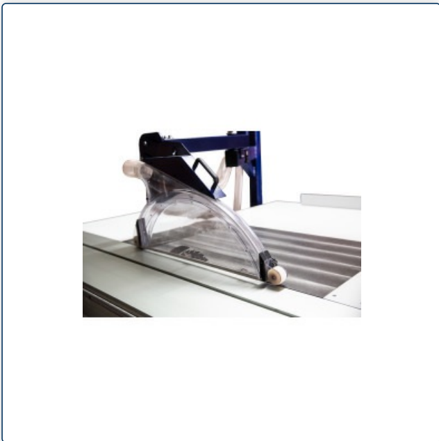
Große Pendelschutzhaube bequem mithilfe einer Gasdruckfeder leicht positionierbar
