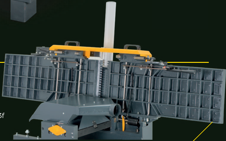
Parallel hinged planing tables Parallelaufklappbare Abrichttische
