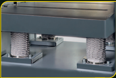
Four-point table fixation – R/F on four screws Dickentisch auf vier Schrauben gelagert
