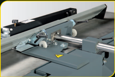
Tilting fence Abrichtanschlag schwenkbar
