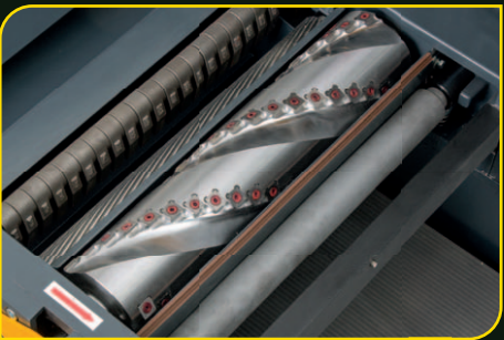
Spiral cutterblock with feeding rollers Spiralmesserwelle mit Vorschubrollen
